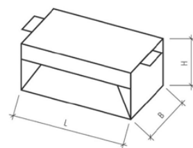
Figura 1: Disegno tecnico
