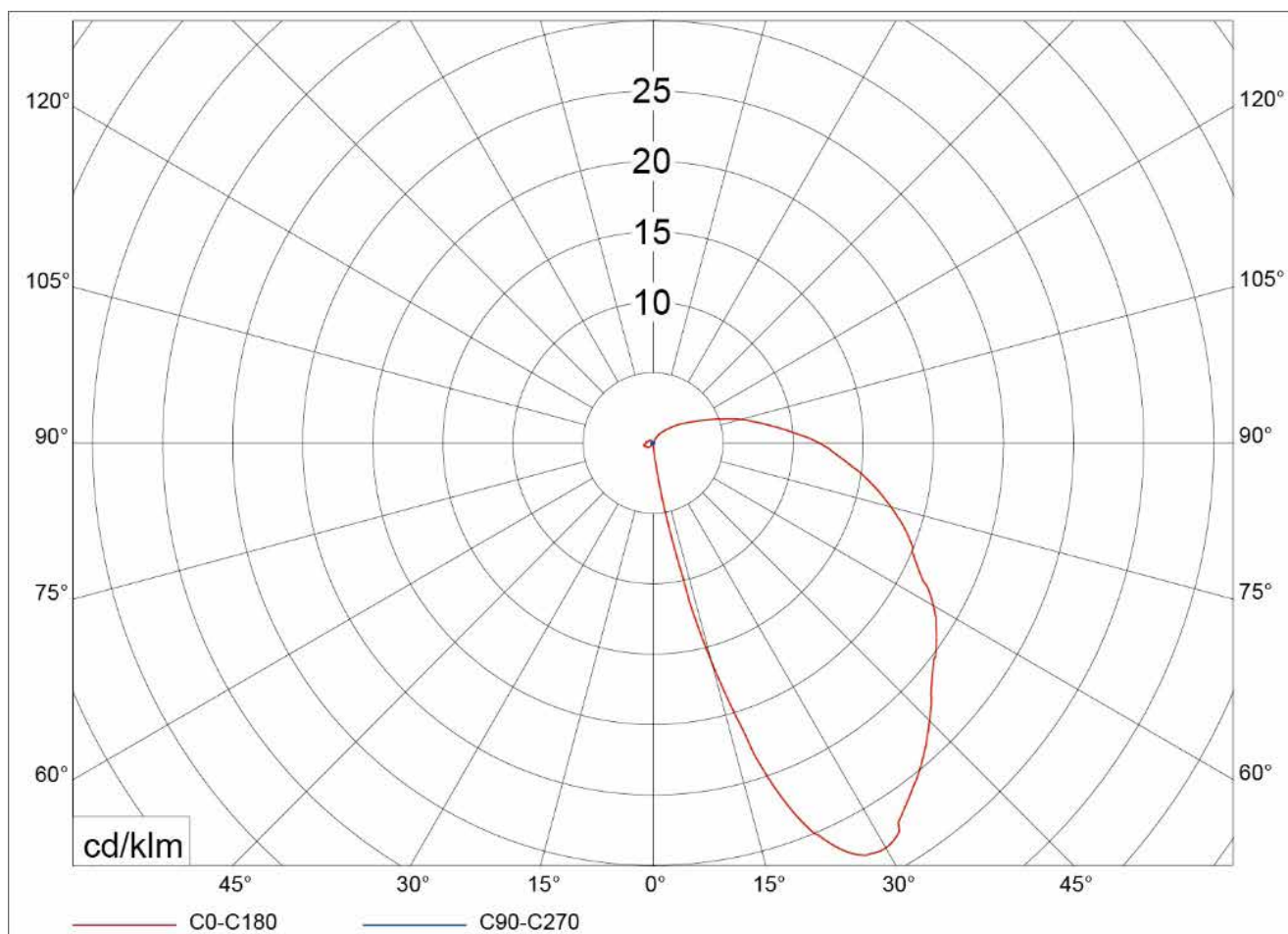
Figura 2: Curva di distribuzione luminosa (LVK)
