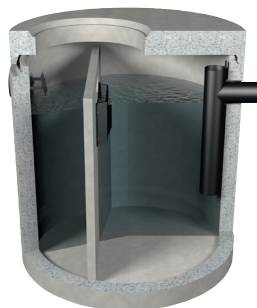
Impianto compatto SFF/FA
