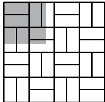
MANHATTAN Platten Verlegemuster 6 5.56 Platten 60/30 pro m 2 Blockverband
