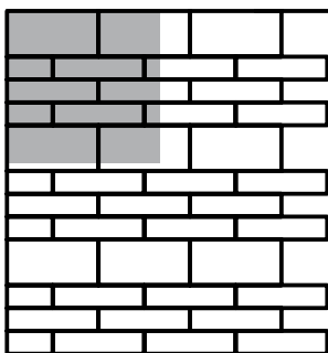
MANHATTAN Platten Verlegemuster 7 2.22 Platten 60/30 pro m 2 6.66 Platten 60/15 pro m 2
