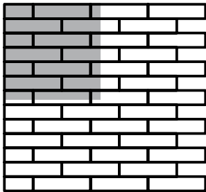
MANHATTAN Platten Verlegemuster 1 11.1 Platten 60/15 pro m 2 Platten 30/15 für die Randausbildung gefräst
