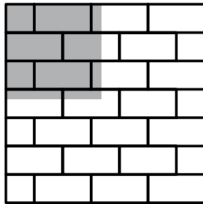
MANHATTAN Platten Verlegemuster 2 5.55 Platten 60/30 pro m 2 Platten 30/30 für die Randausbildung gefräst
