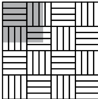
MANHATTAN Platten Verlegemuster 5 11.1 Platten 60/15 pro m 2 Blockverband
