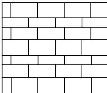
B Verband 1/3 zu 2/3
