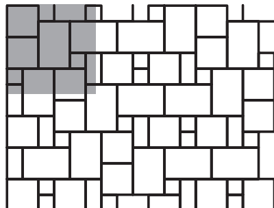
Verlegemuster 1
