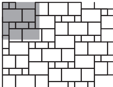
Verlegemuster 2
